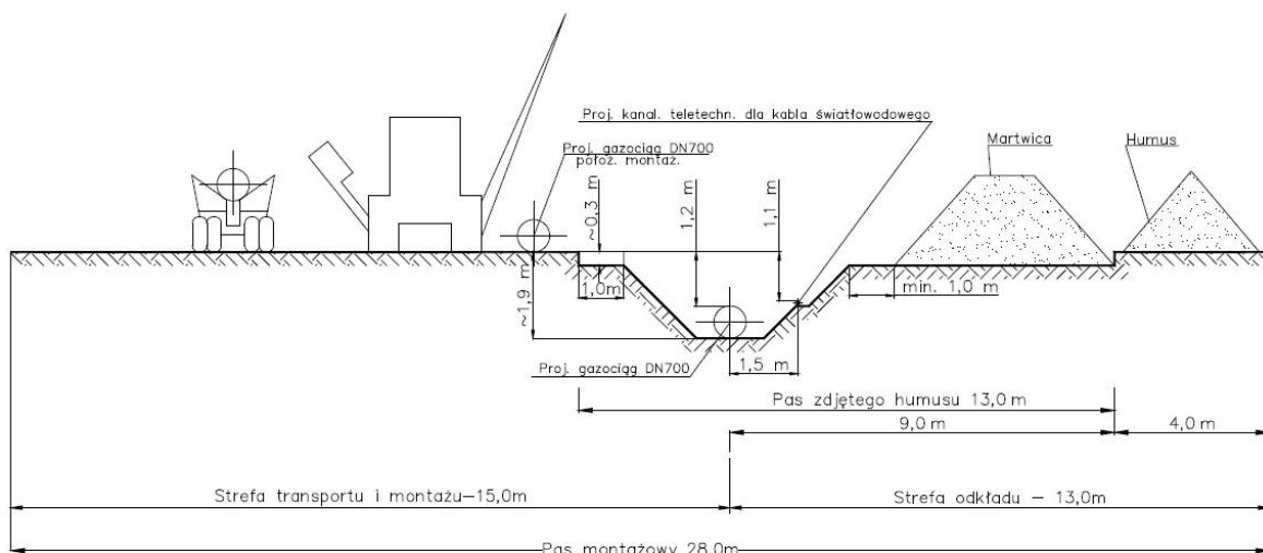
Rys. 3. Poglądowy schemat zagospodarowania pasa montażowego w trakcie budowy - tereny rolne
